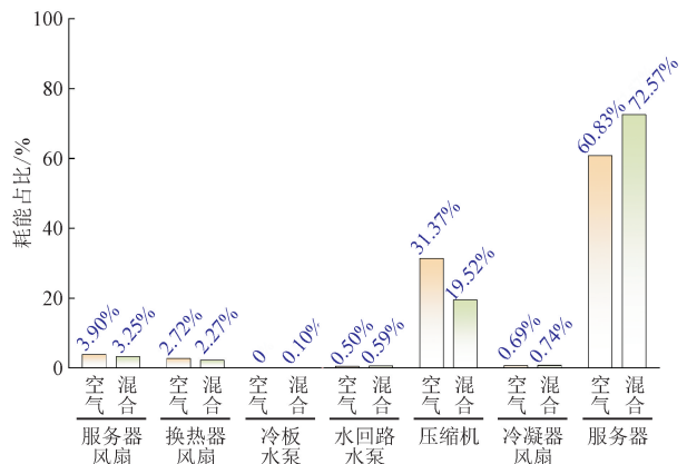
图 12 两种冷却方式下冷却系统各部件能耗的占比
