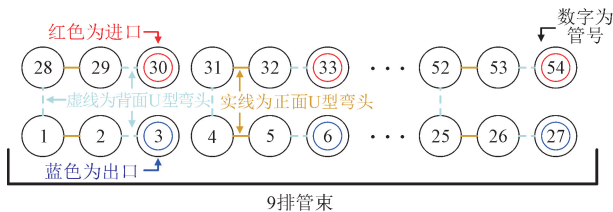
图 5 空气-水换热器管束结构
