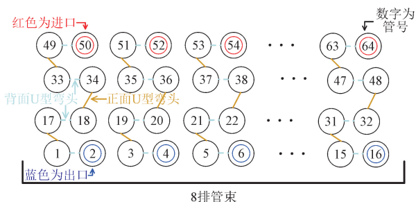
图 7 冷凝器管束结构
